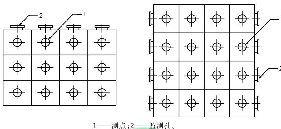
图4 矩形断面测点与监测孔示意图
