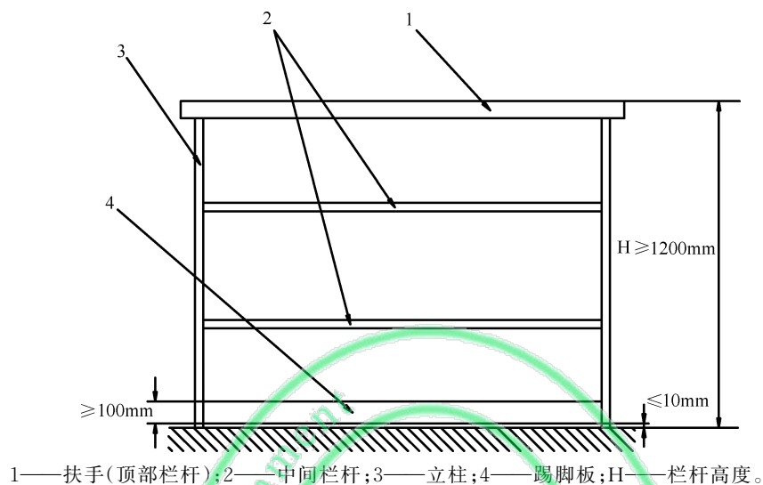
图 5 防护栏杆示意图
