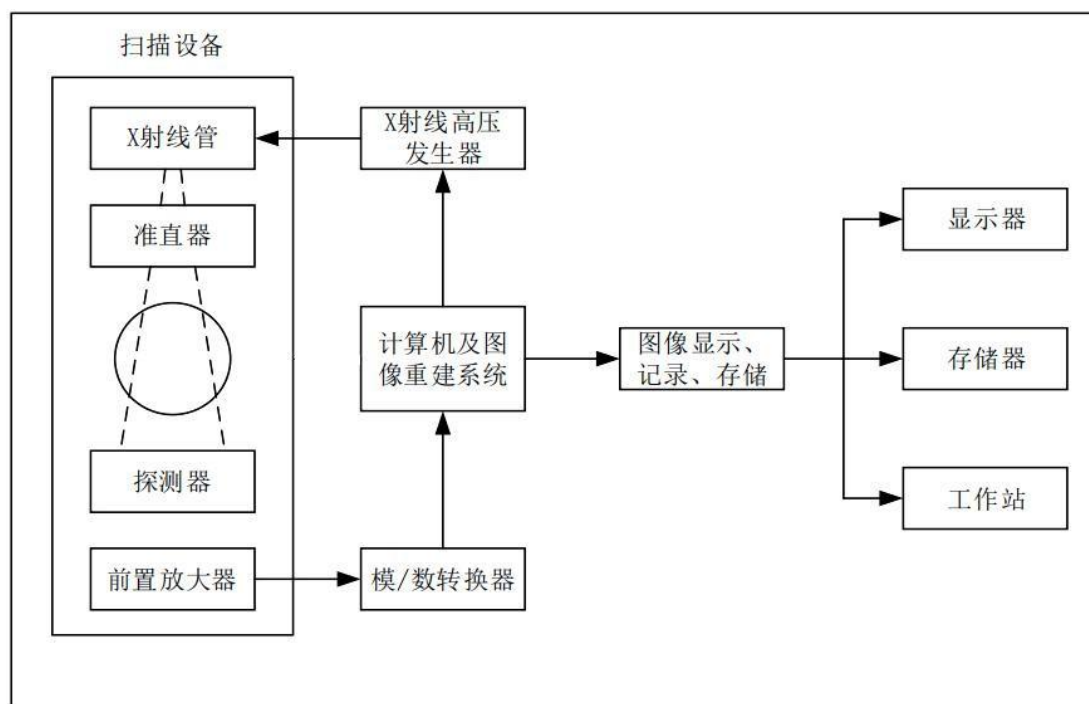
图 9.1-1 工业快速 CT 机系统组成示意图
