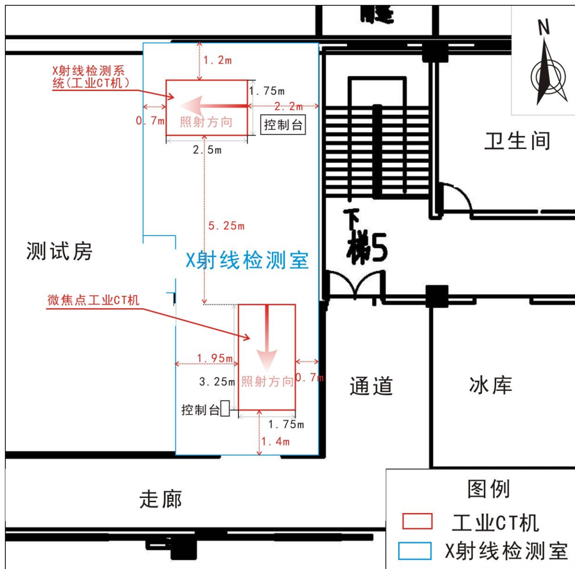
图 7-2 X 射线检测室平面布局示意图
