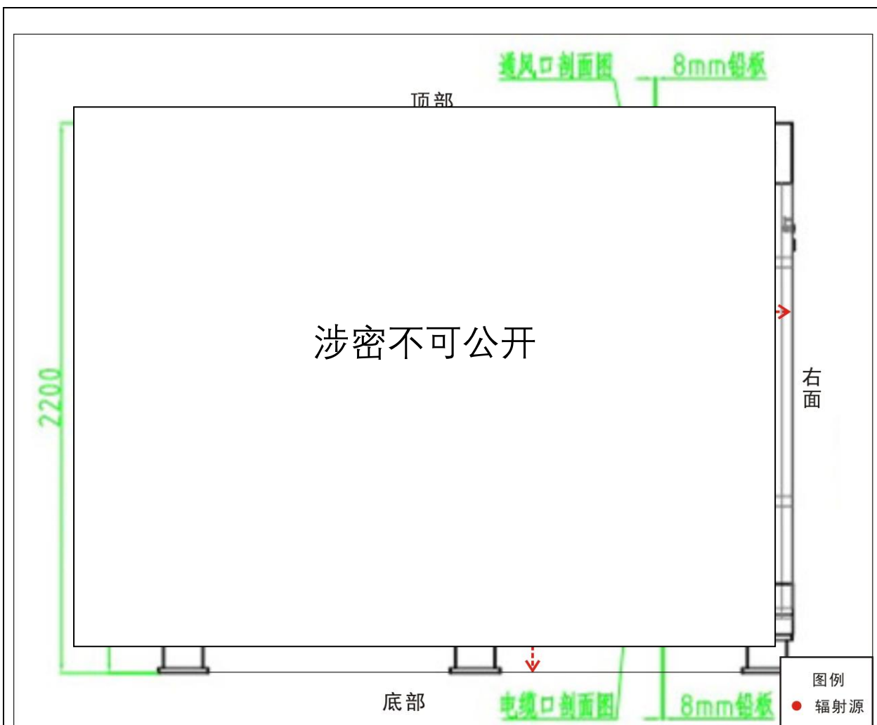
图 11-2 X 射线检测系统辐射源点距四周屏蔽体外表面距离示意图（正视图）
