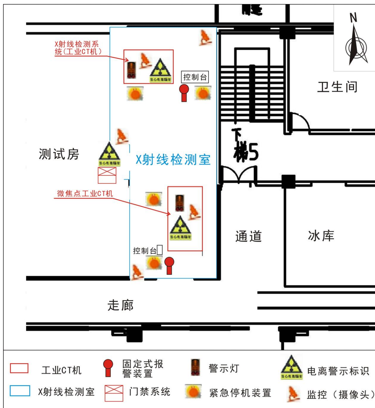
图 10-4 辐射安全设施设置示意图
