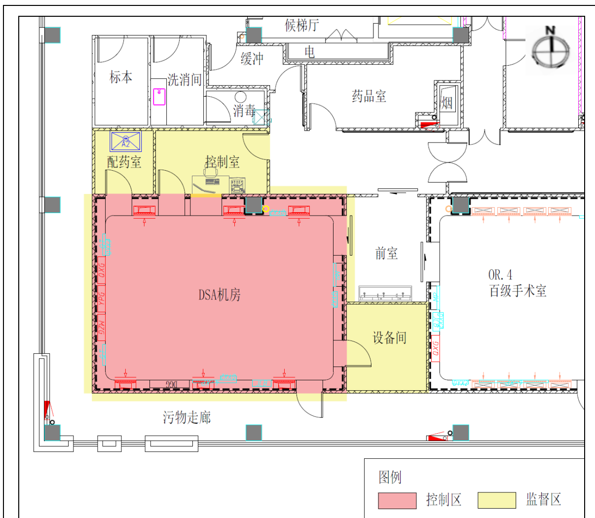
图 10-1 本项目 DSA 机工作场所分区示意图
