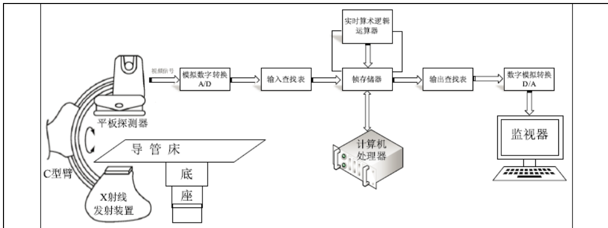
图 9-2 平板探测器型 DSA 机系统结构图
