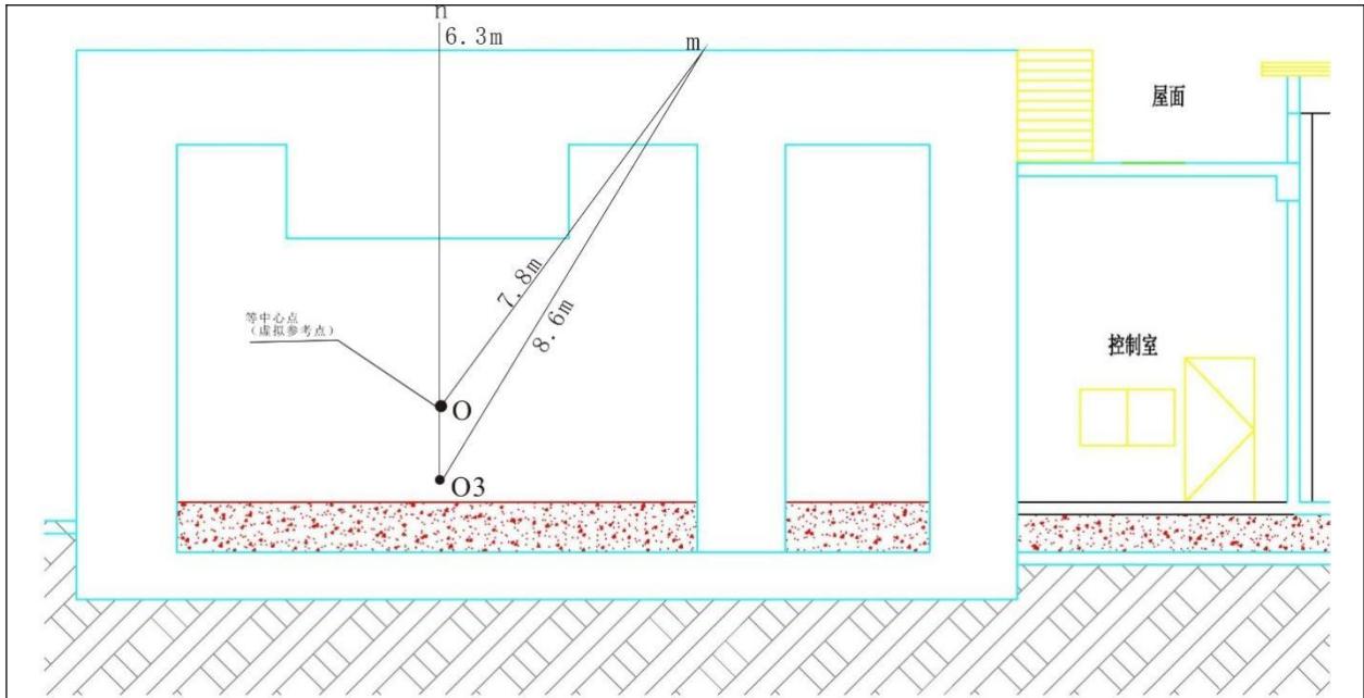
图 11-2 直线加速器机房关注点分布图（剖面）
