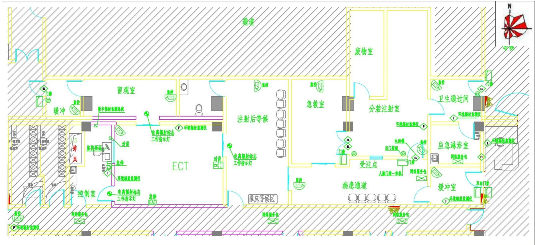
图 10-5 核医学科辐射安全防护设施设备设置位置示意图
