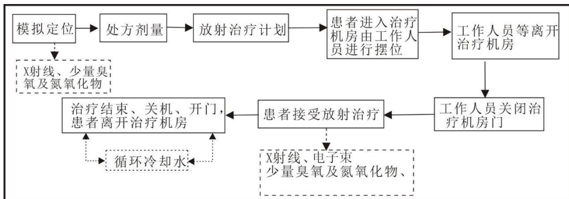
图 9-2 直线加速器工艺流程及产污环节示意图
