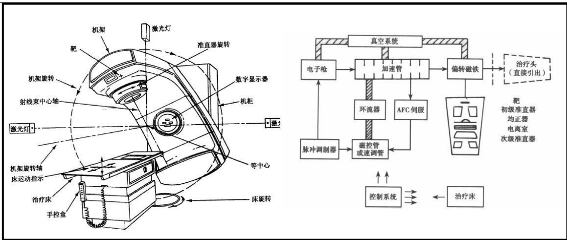
图 9-1 医用电子直线加速器物理结构图（左）及内部结构图（右）
