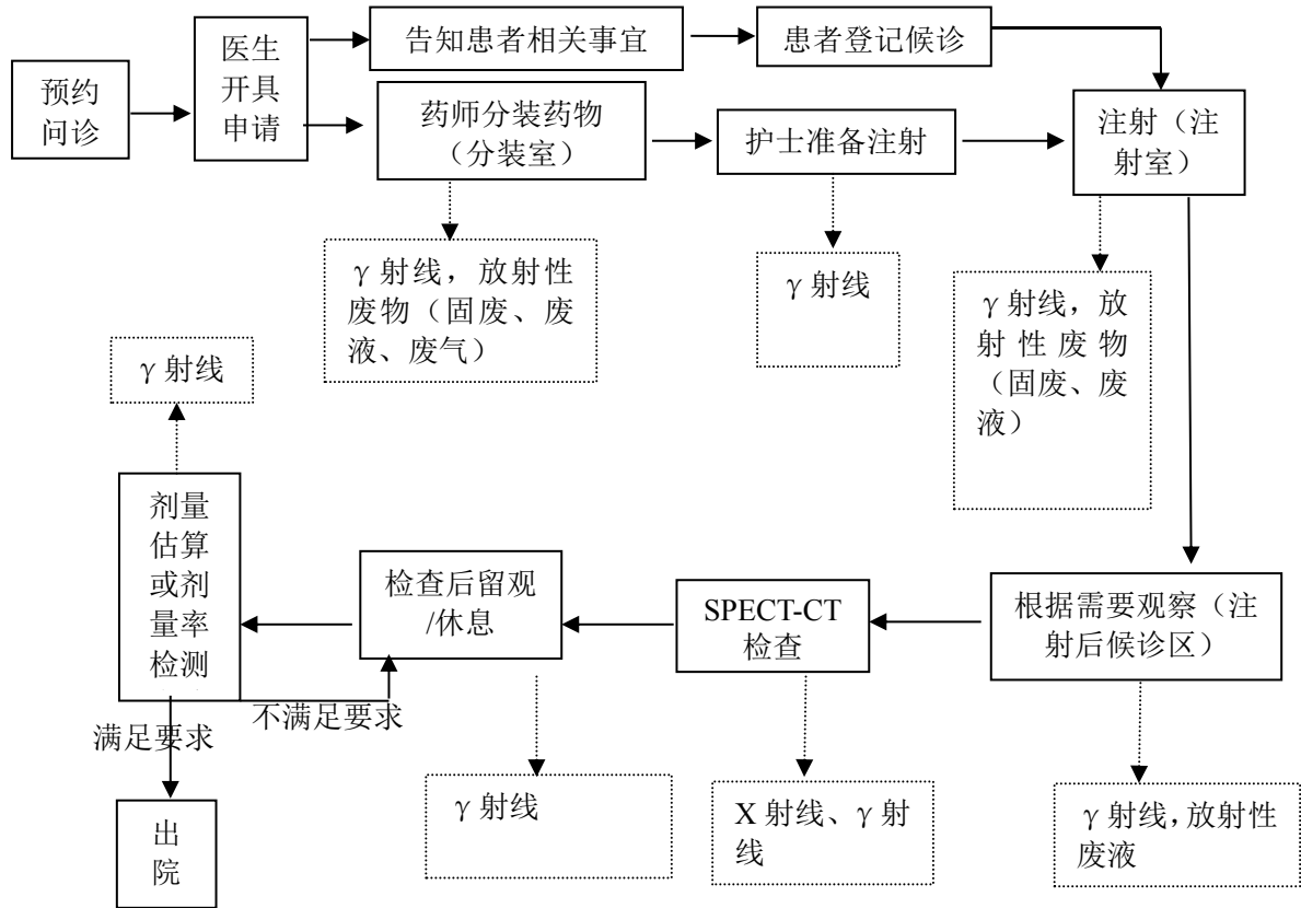
图 9-4 SPECT 检查工艺流程及产污环节示意图
