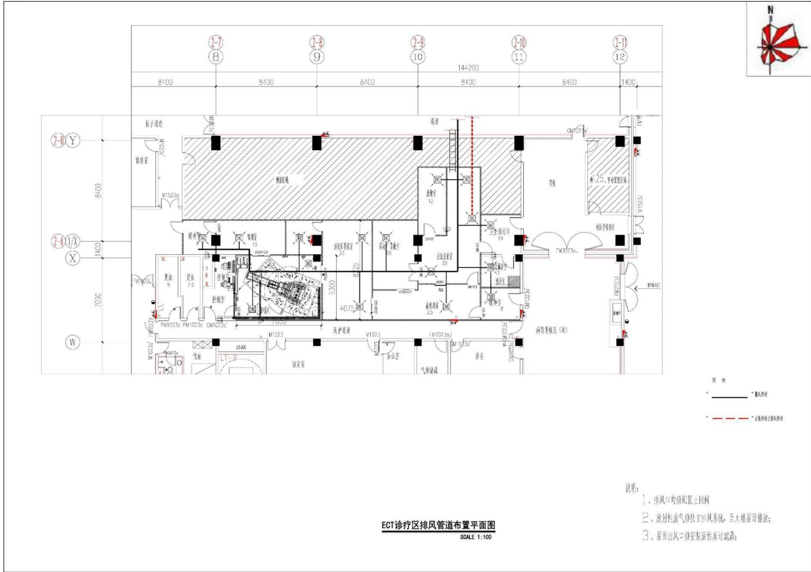
图 10-6 核医学科排风管道路线图
