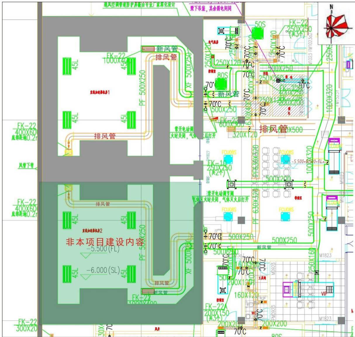
图 10-4 直线加速器机房排风管道路线图
