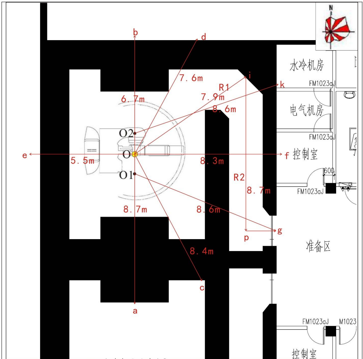
图 11-1 直线加速器机房关注点分布图（平面）
