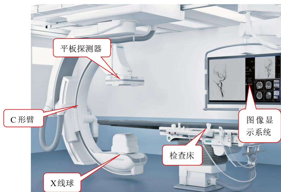
图 9-1 Artis Q Ceiling 型 DSA 机外观示意图
