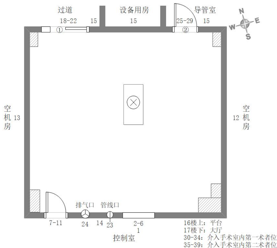
图11.2-5 类比对象检测点位示意图
