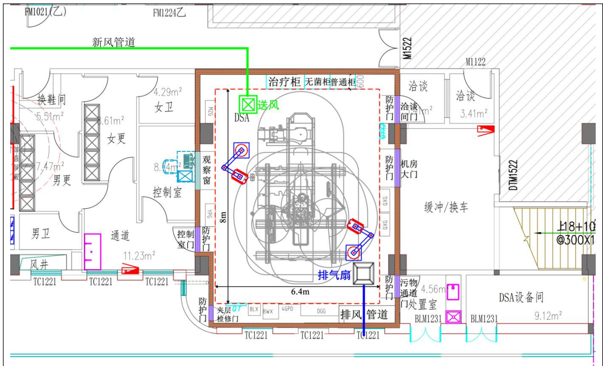
图10.1-6 新风和排风管道示意图
