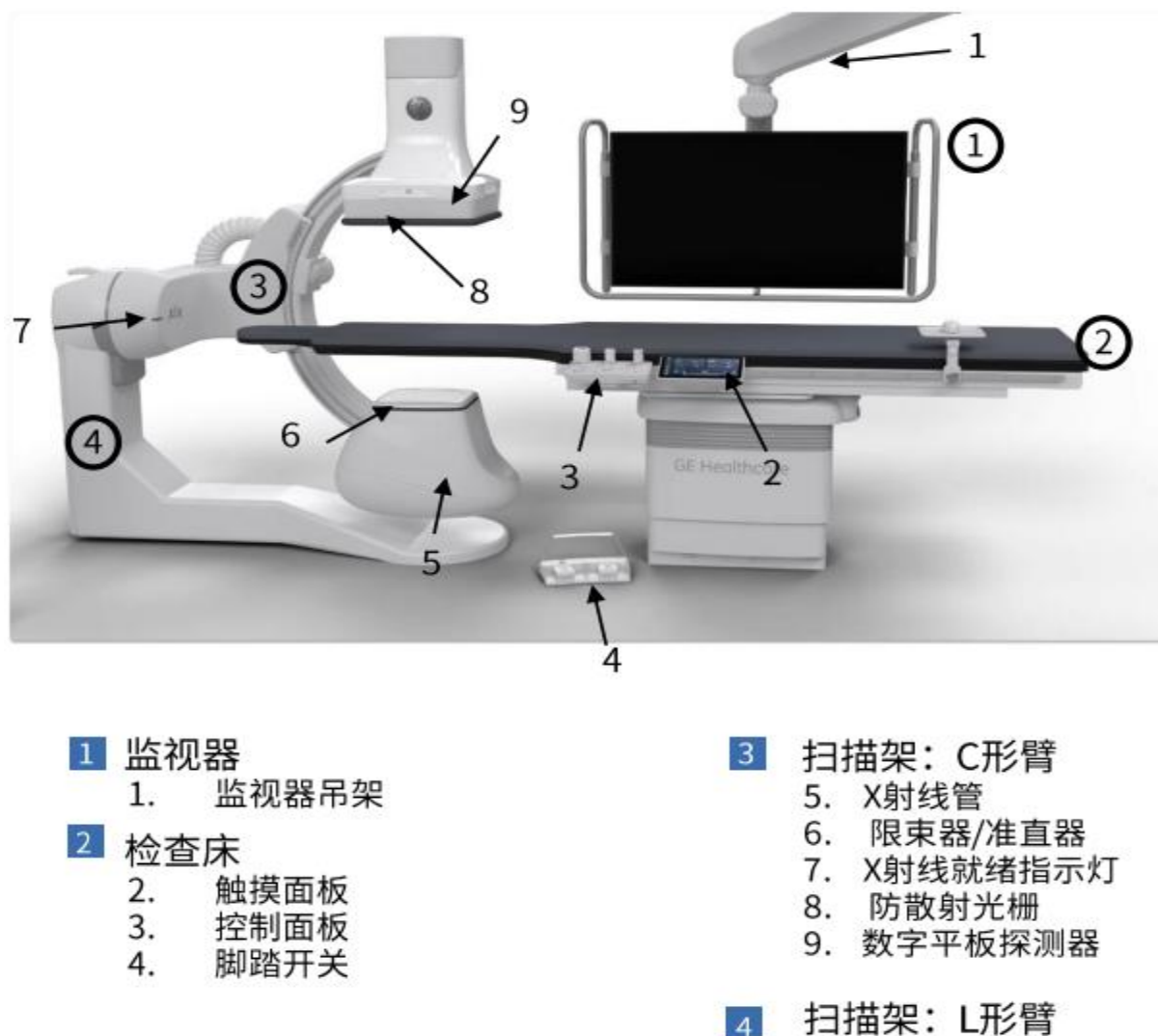
图9.1-1 DSA设备外观示意图
