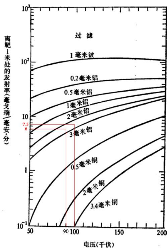
图 11.2-1 离靶1m处的发射率常数随管电压及总滤过厚度变化的情况
