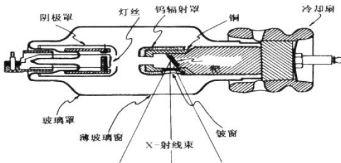
图9.1-2 典型X射线管结构图
