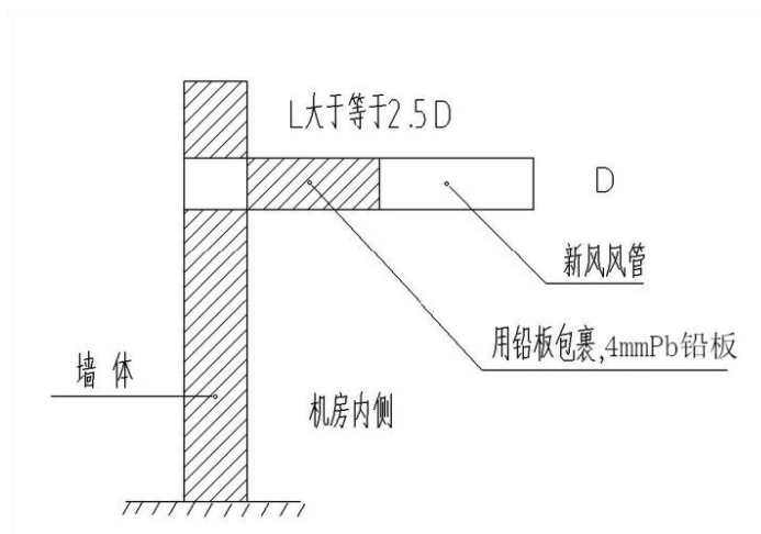
图10.1-5 风管穿墙防护示意图
