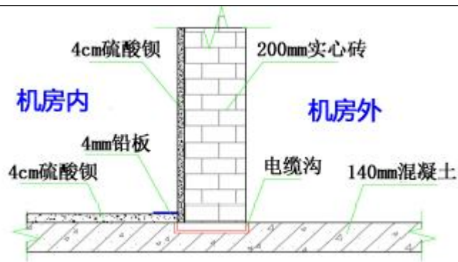
图10.1-4 电缆沟穿墙线管防护示意图
