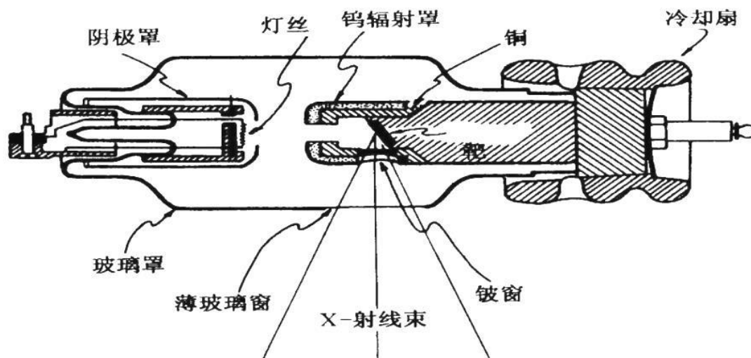
图 9-3 X 射线管结构示意图
