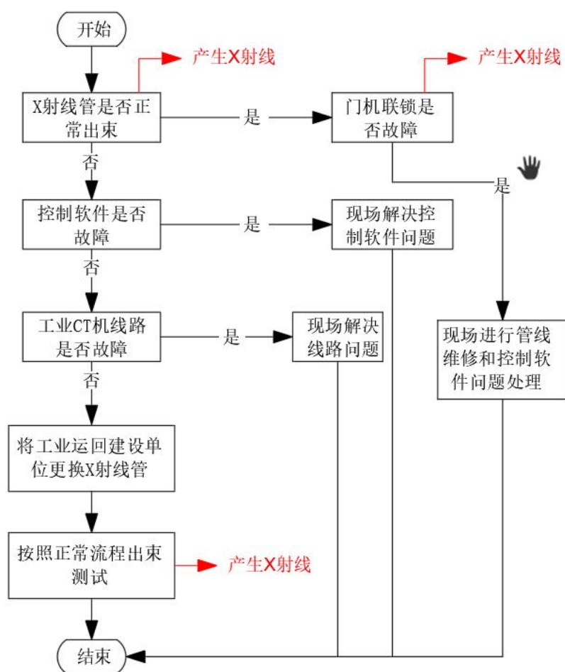
图 9-6 工业 CT 维修流程及产污环节图
