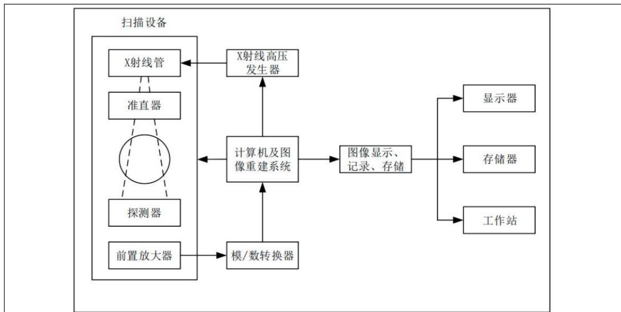
图 9-2 本项目工业 CT 机组组成示意图
