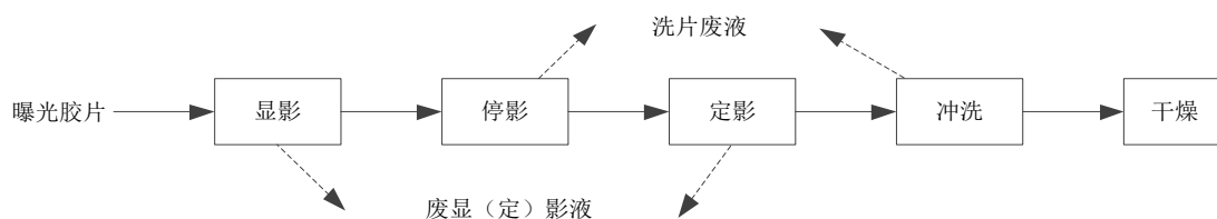
图 9-7 洗片工艺流程及产污环节示意图
