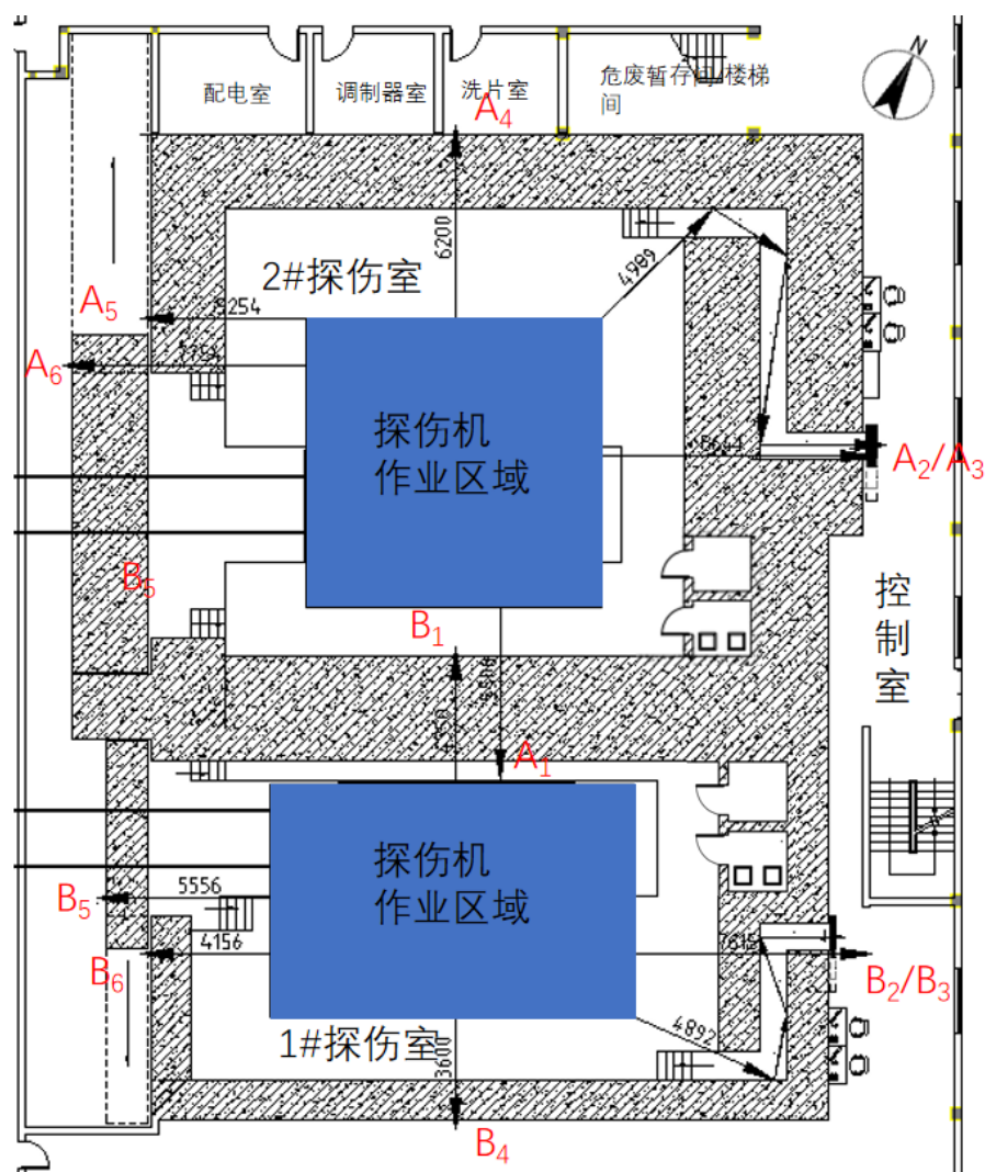
图 11-2 \gamma 射线探伤机预测点位平面示意图 (单位: mm)
