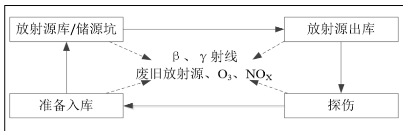
图 9-5 放射源暂存库/储源坑工作及产污流程示意图
