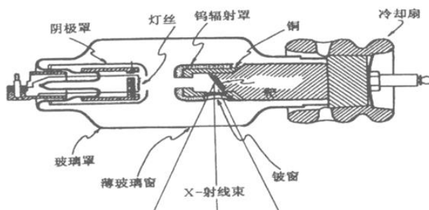
图 9-9 典型 X 射线管结构图
