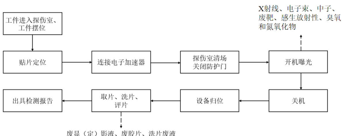
图 9-12 电子直线加速器探伤工艺流程及产污环节示意图
