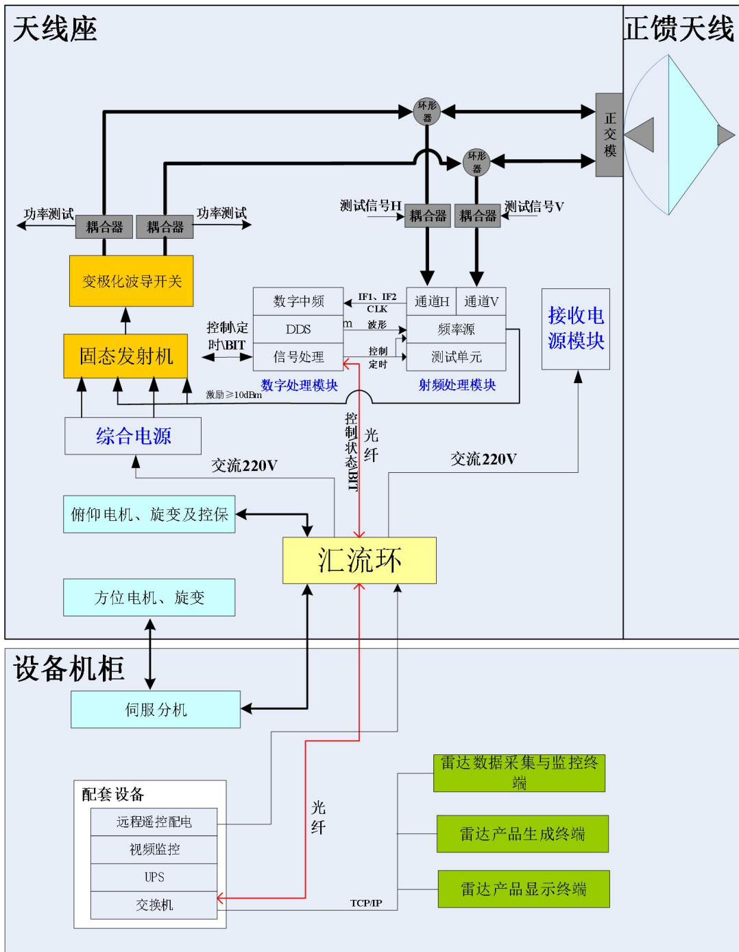
图 5.1-2 X 波段双偏振天气雷达工作原理框图
