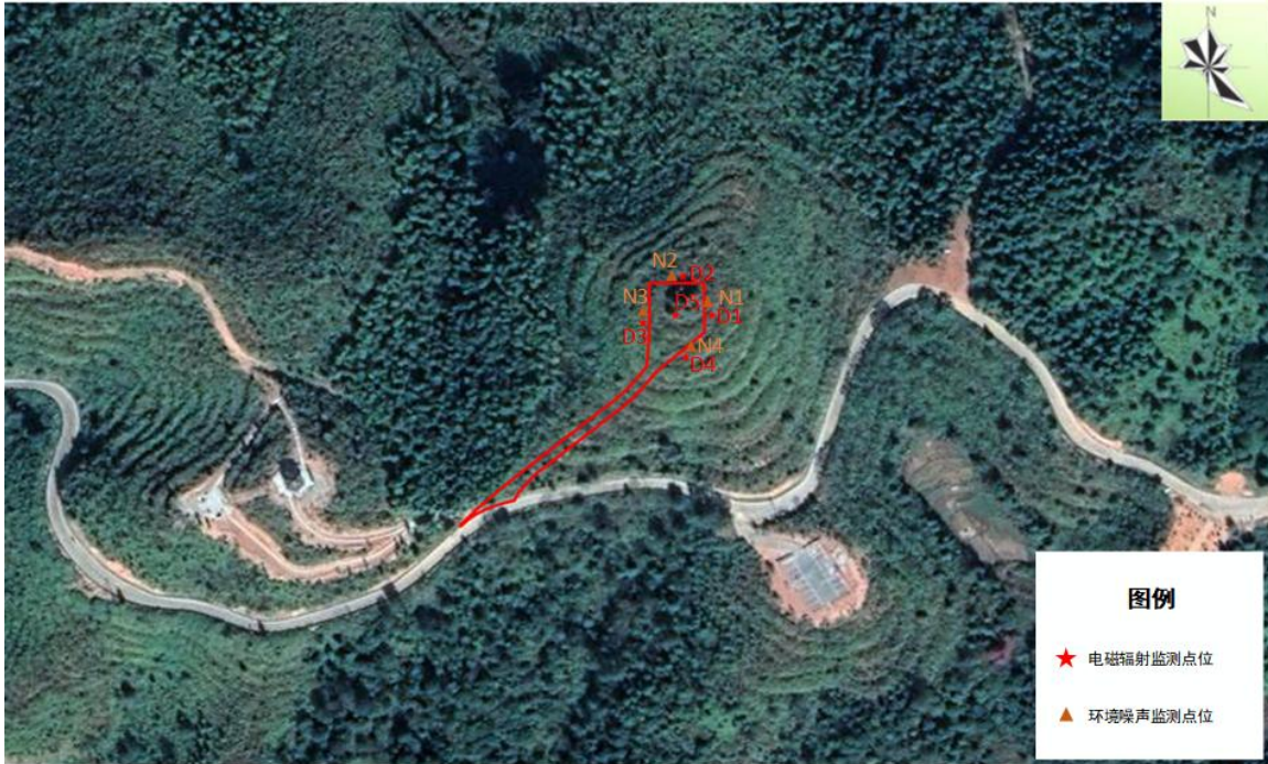
图 3.6-1 噪声环境监测点位图
