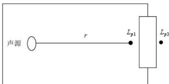
图 6.2-1 室内声源等效为室外声源图例
