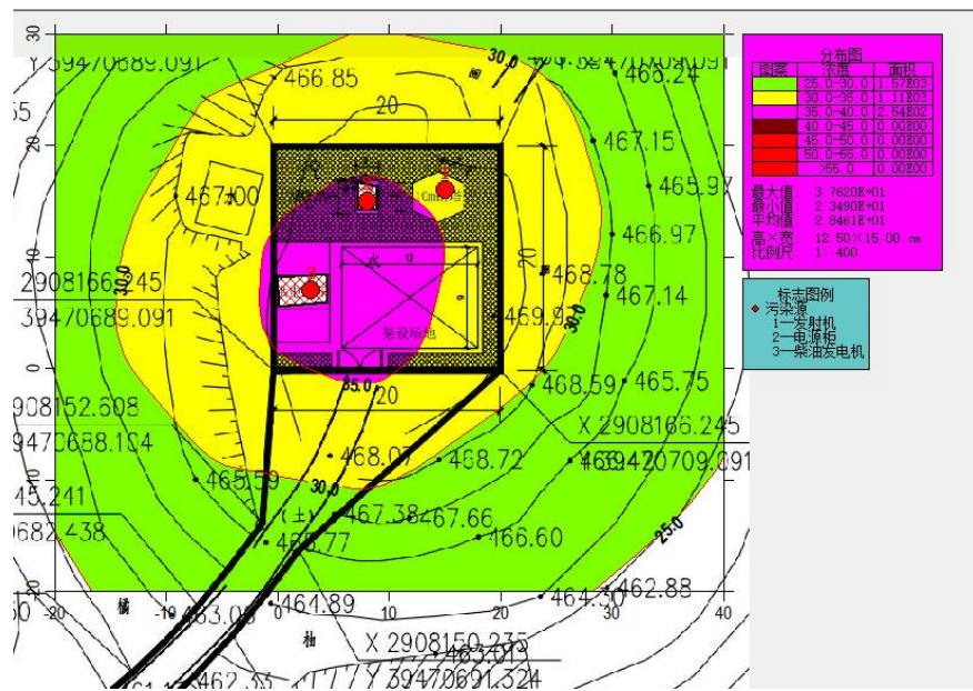
图 6.2-2 噪声贡献值预测分布图
