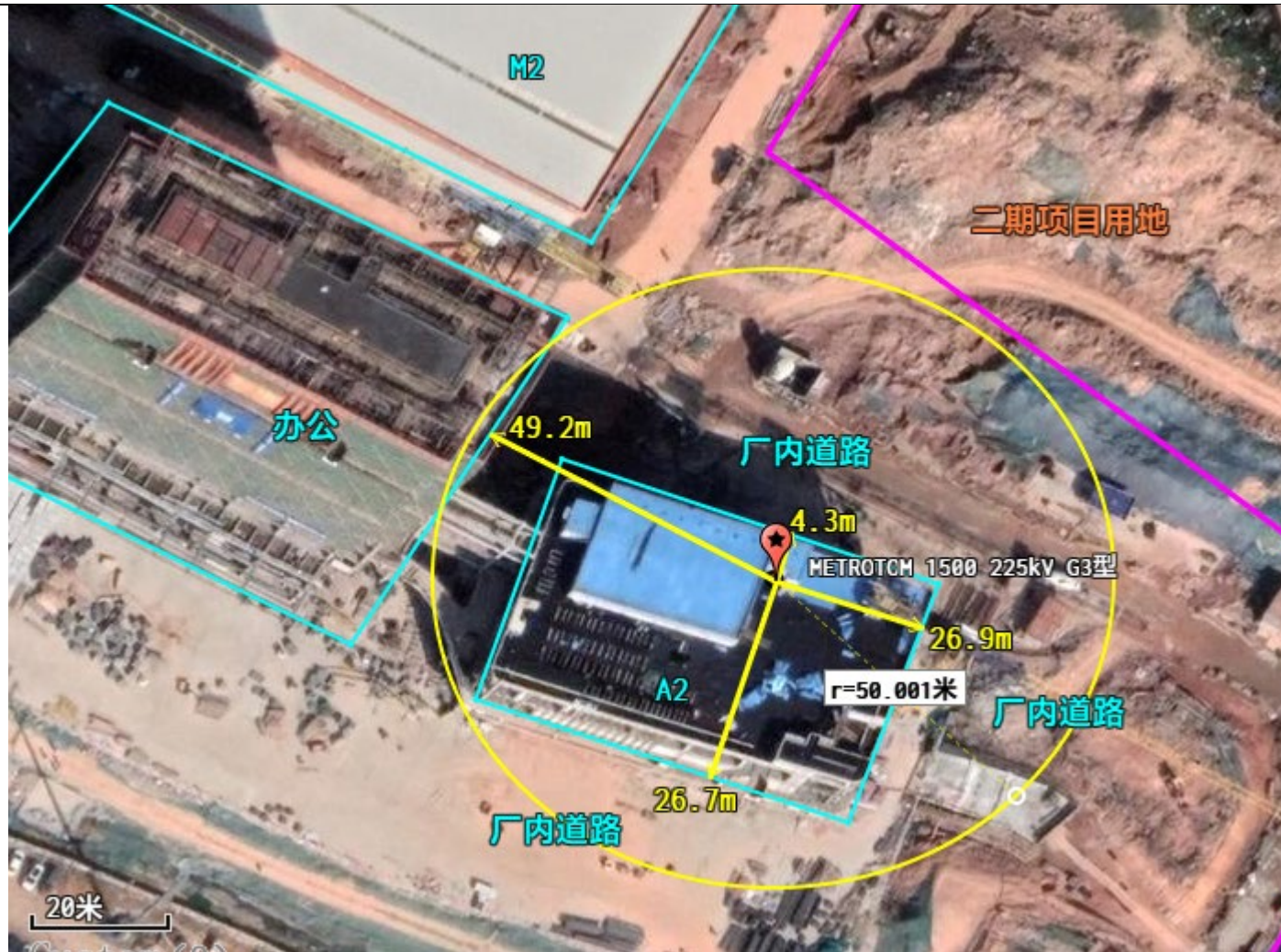
图 1.4 METROTOM 1500 225kV G3 型工业 CT 机所在厂房四周环境示意图
