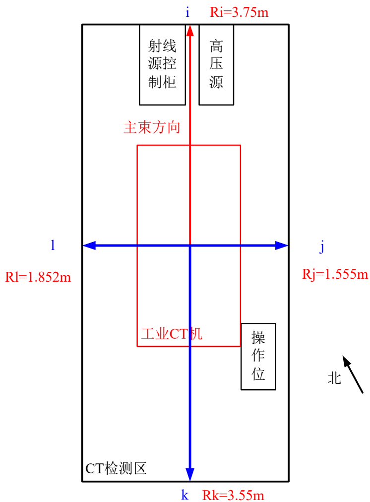
图 11.6 参考点及辐射路径示意图（CT 检测区平面）
