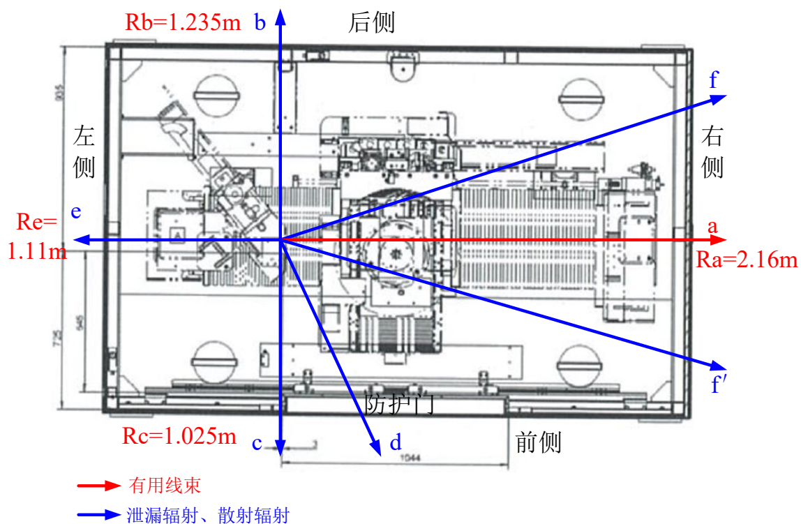
图 11.1 参考点及辐射路径示意图（俯视透视）
