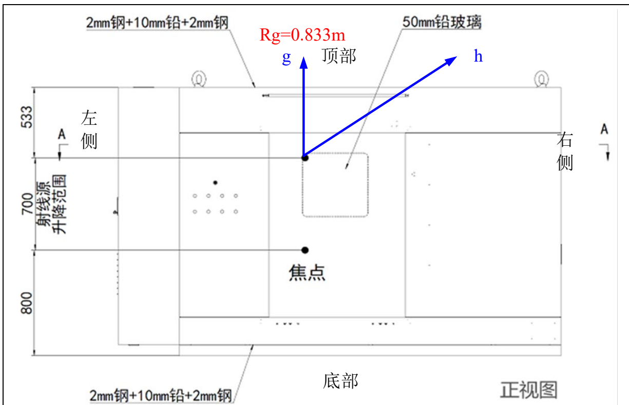
图 11.5 参考点及辐射路径示意图（面向设备透视）
