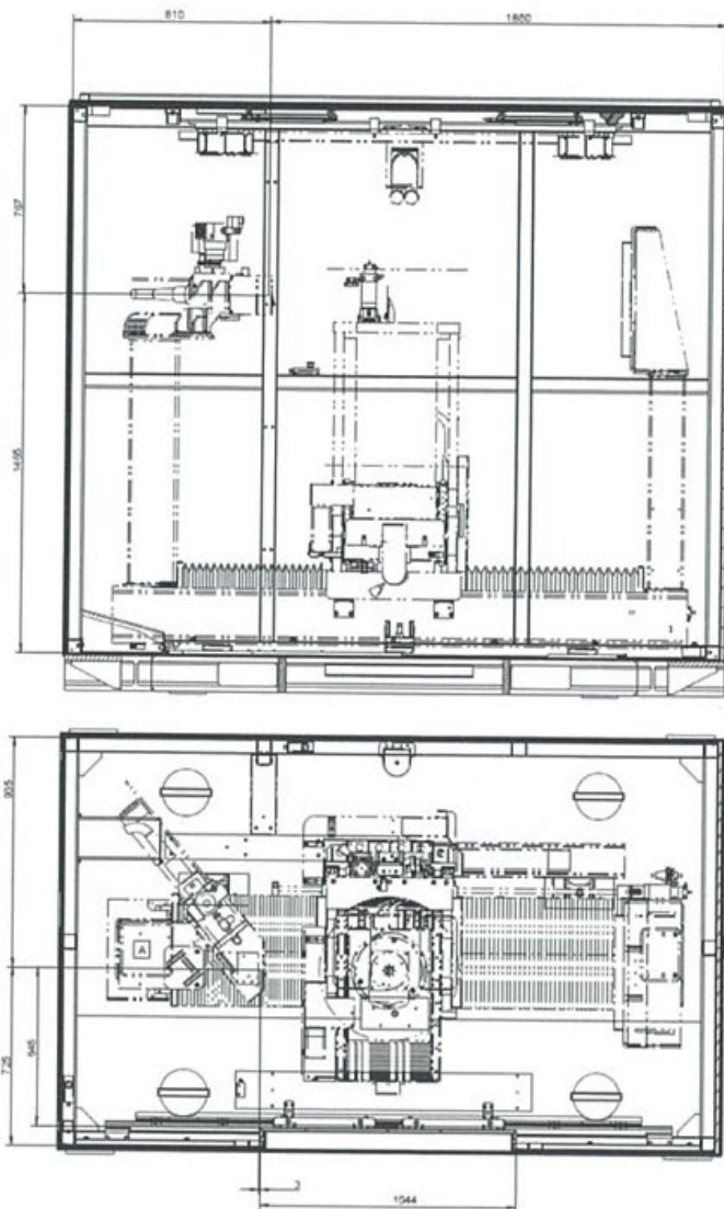
图 9.3 项目 METROTOM 1500 225kV G3 型工业 CT 机结构示意图
