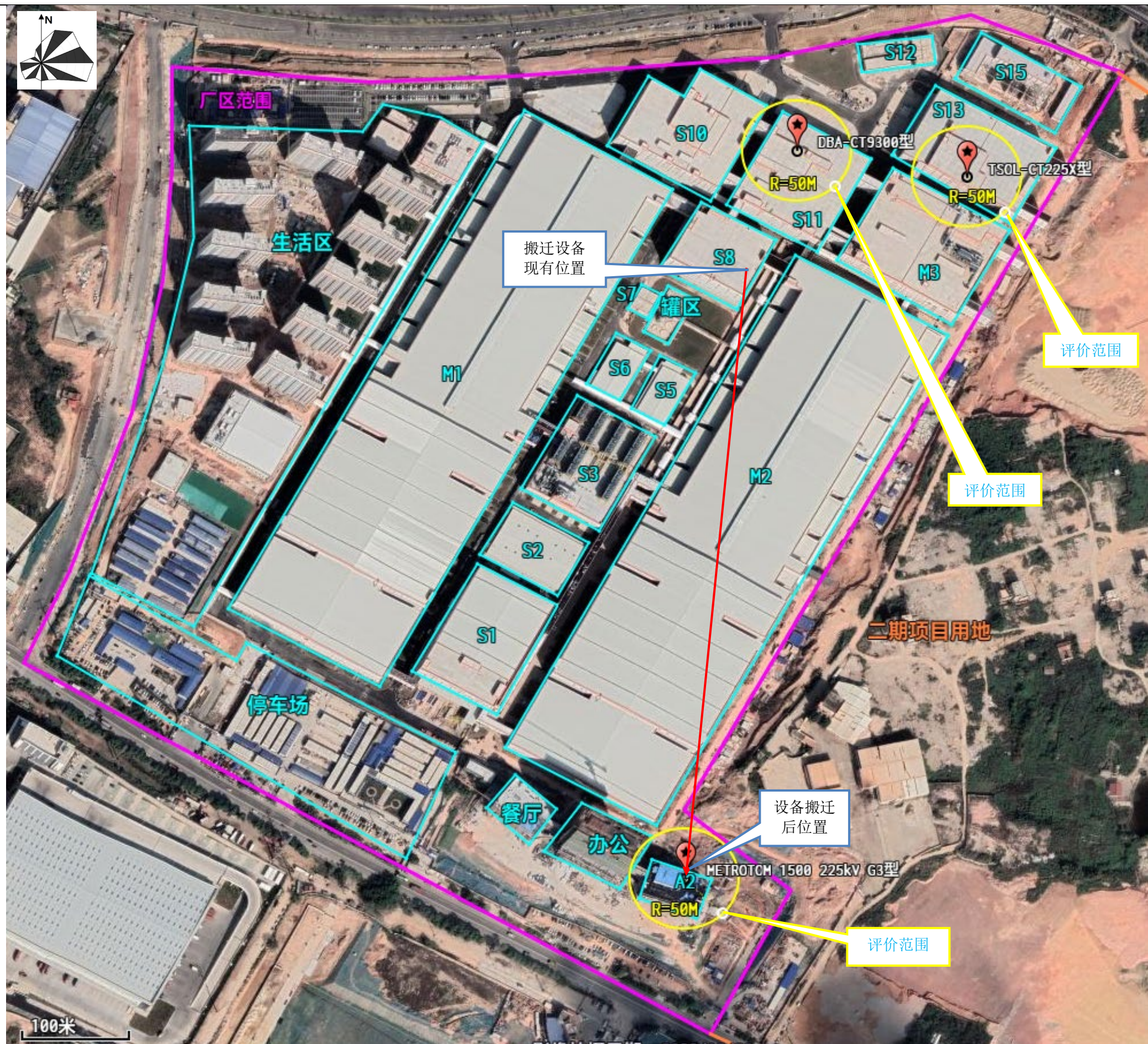
图 1.3 厦门新能安科技有限公司总平面布置及评价范围示意图
