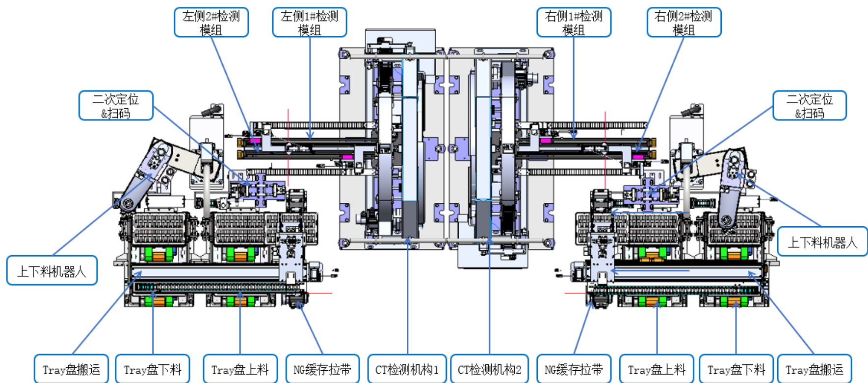
图 9.10 项目 DBA-CT9300 型工业 CT 机布局平面示意图
