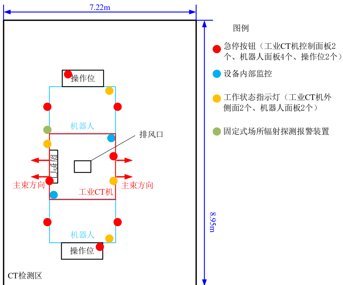
图 10.6 S11 四层 CT 检测区防护装置示意图
