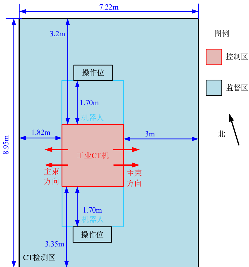
图 10.2 S13 一层 CT 检测区控制区与监督区划分图
