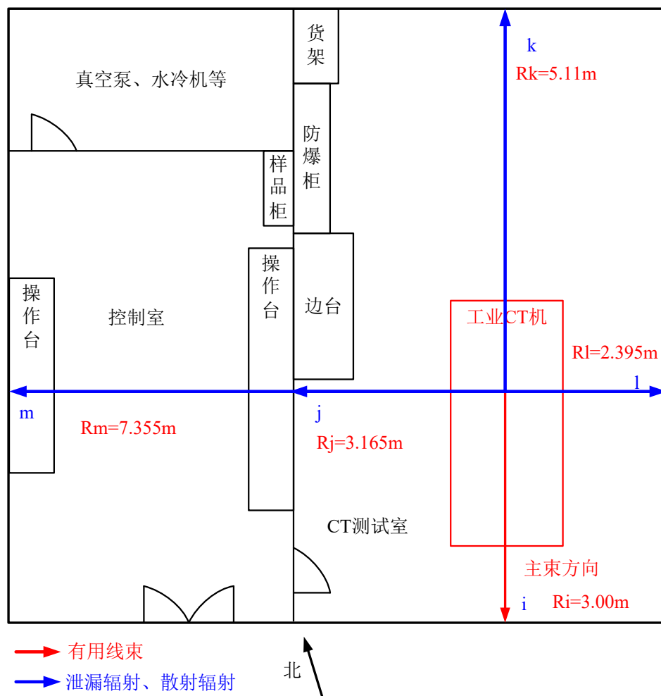
图 11.3 参考点及辐射路径示意图（CT 测试室平面）
