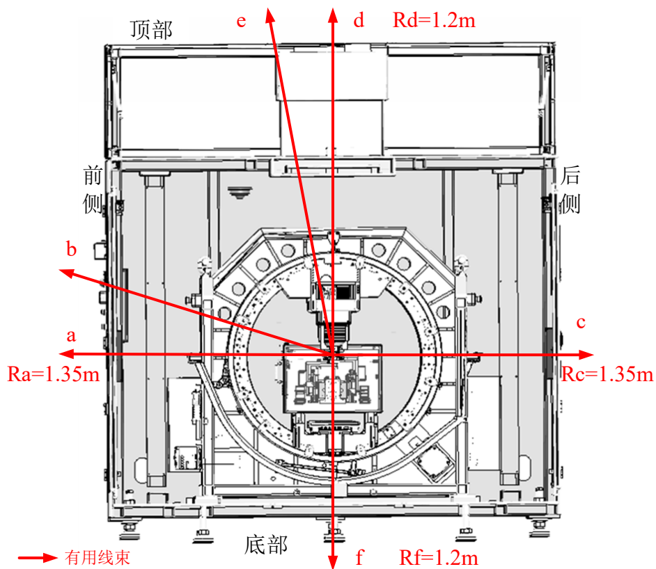
图 11.8 参考点及辐射路径示意图（设备左侧面透视）
