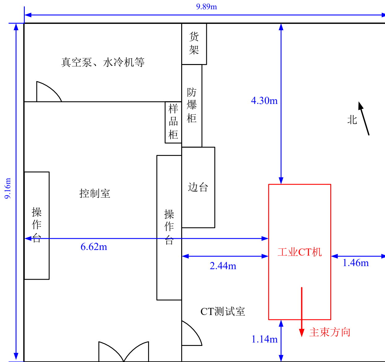
图 1.7 A2 一层 CT 测试室平面布置图（CT 测试室为单独隔间，四周均有实体墙体）
