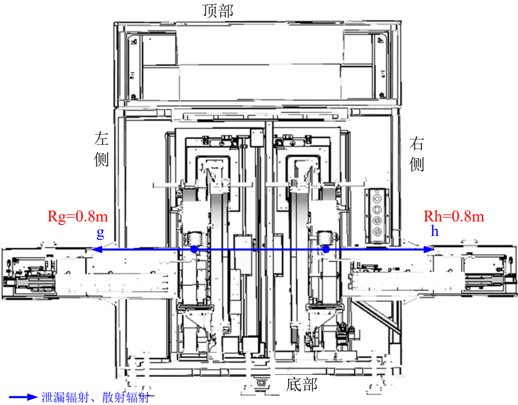
图 11.7 参考点及辐射路径示意图（面向设备透视）
