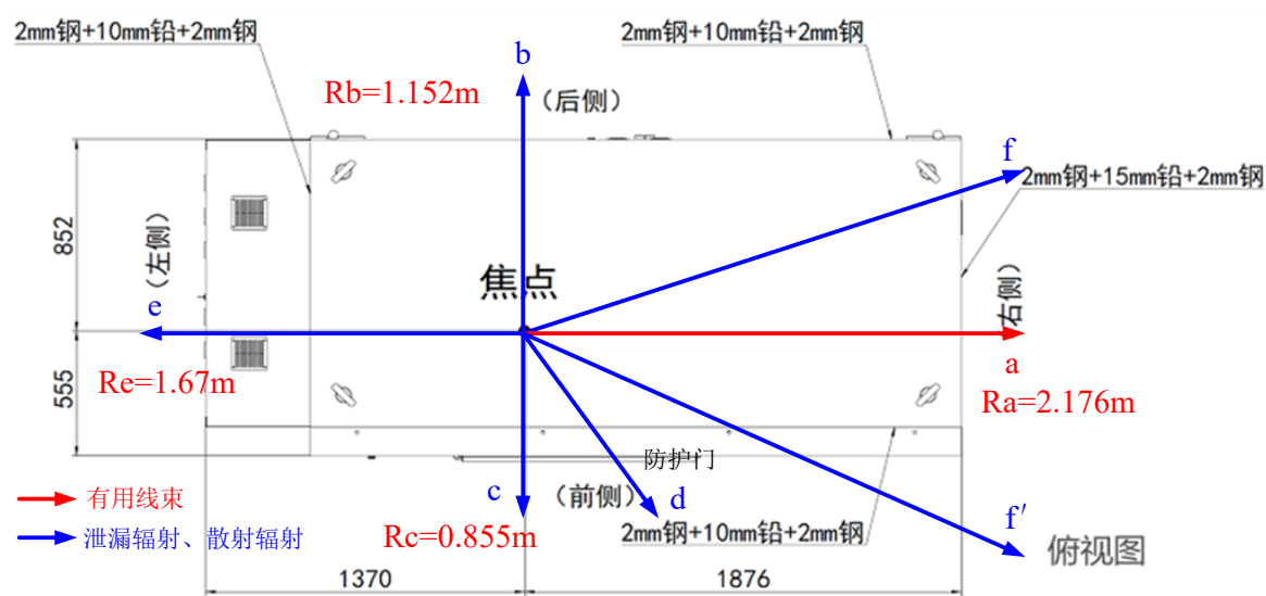
图 11.4 参考点及辐射路径示意图（俯视透视）
