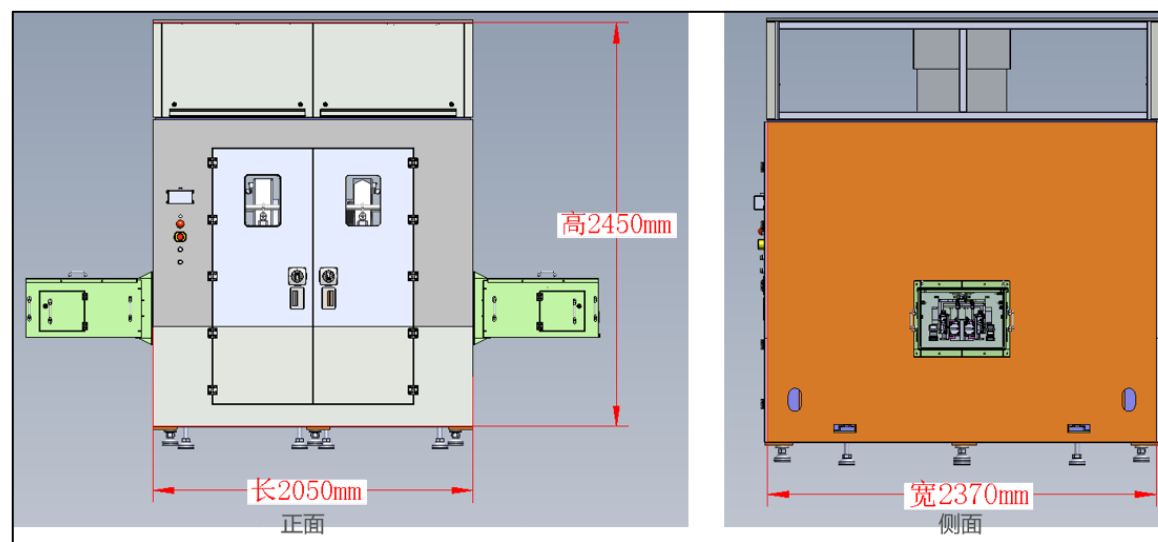
图 9.11 项目 DBA-CT9300 型工业 CT 机结构示意图
