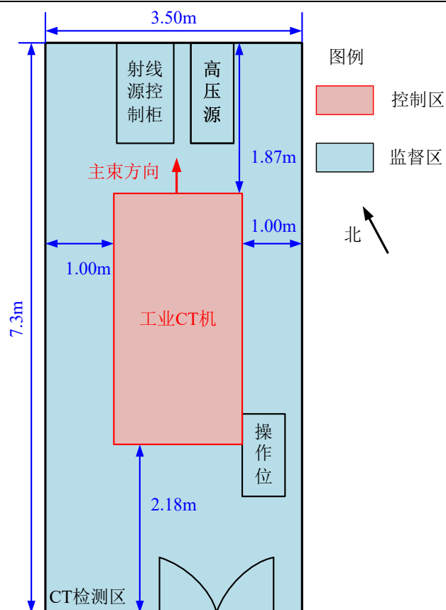
图 10.2 S13 一层 CT 检测区控制区与监督区划分图
