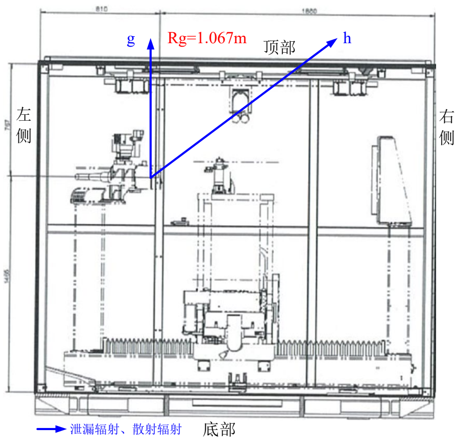
图 11.2 参考点及辐射路径示意图（面向设备透视）
