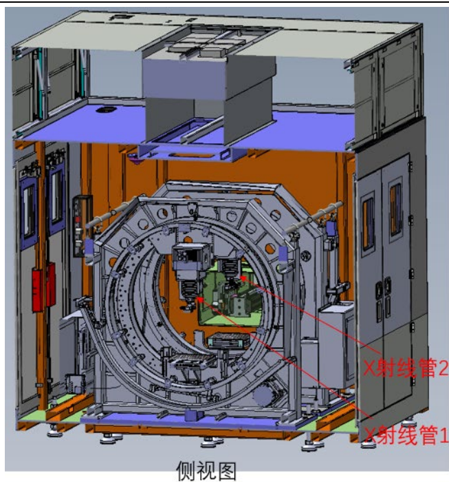
图 9.12 项目 DBA-CT9300 型工业 CT 机结构示意图
