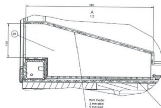
图 9.5 项目 METROTOM 1500 225kV G3 型工业 CT 机结构示意图
