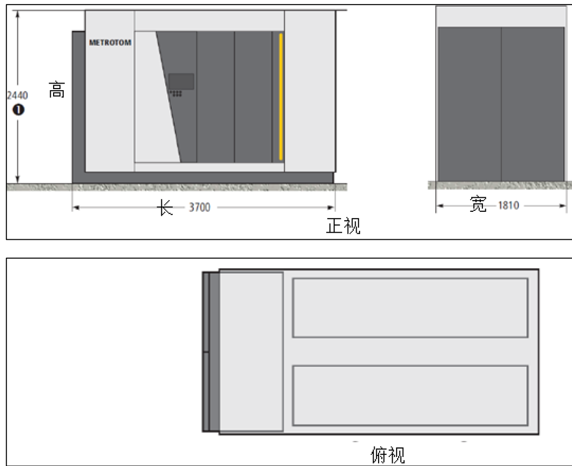
图 9.2 项目 METROTOM 1500 225kV G3 型工业 CT 机结构示意图
