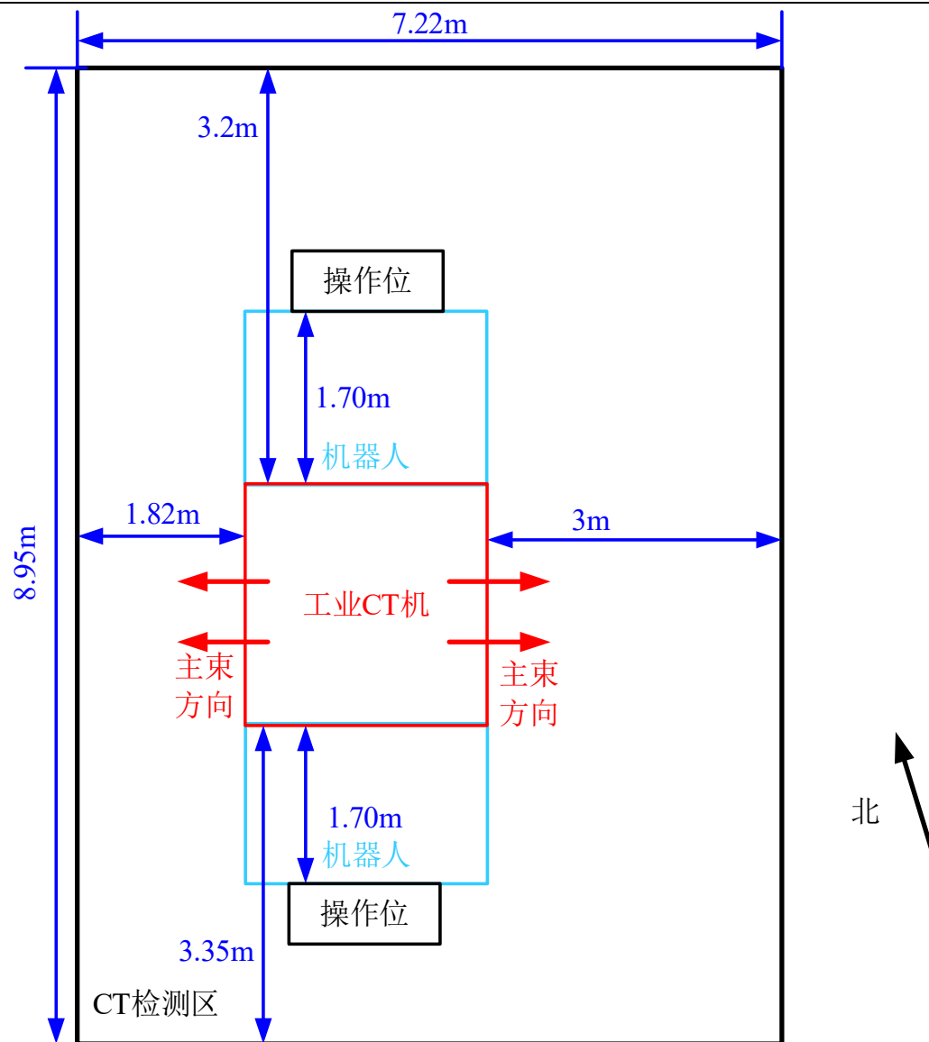
图 1.13 S11 四层 CT 检测区平面布置图 (CT 检测区东侧有实体墙体, 北侧、西侧、南侧为车间内部)
