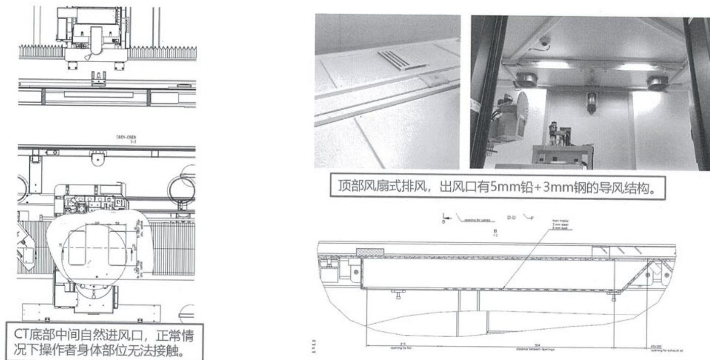
图 9.6 项目 METROTOM 1500 225kV G3 型工业 CT 机结构示意图
