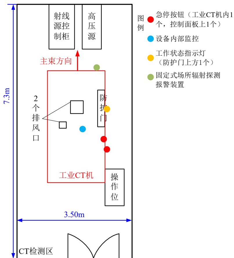
图 10.5 S13 一层 CT 检测区防护装置示意图
