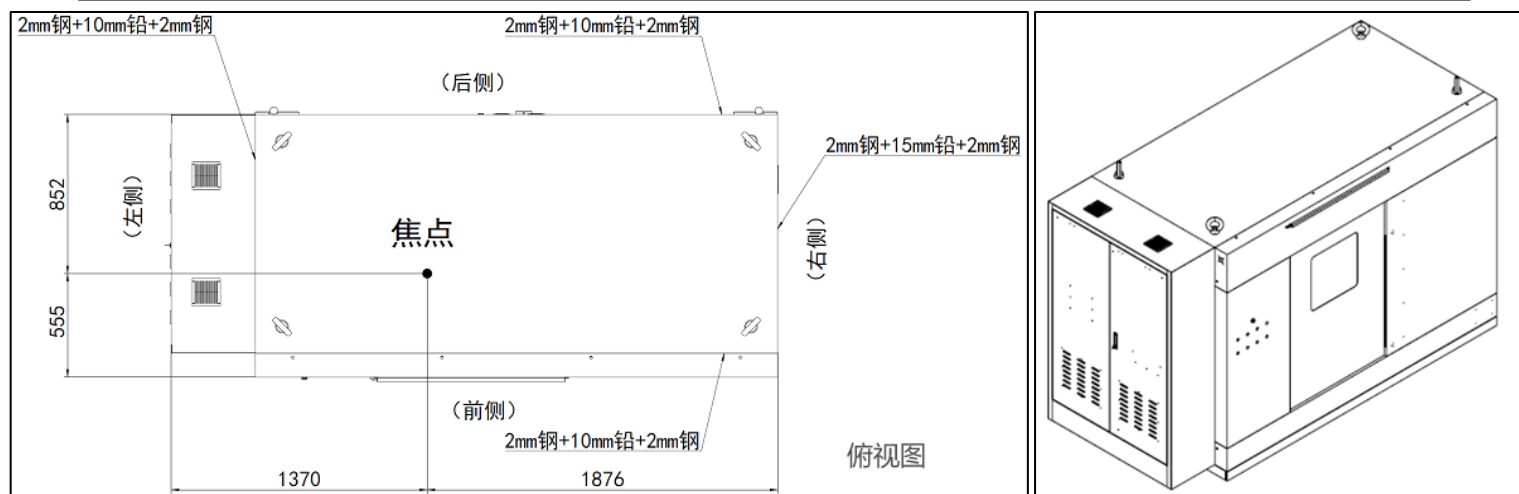
图 9.8 项目 TSOL-CT225X 型工业 CT 机结构示意图
