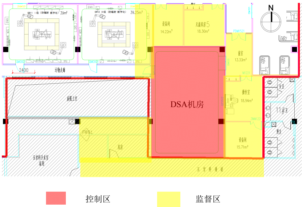
图 10-1 DSA工作场所分区图
