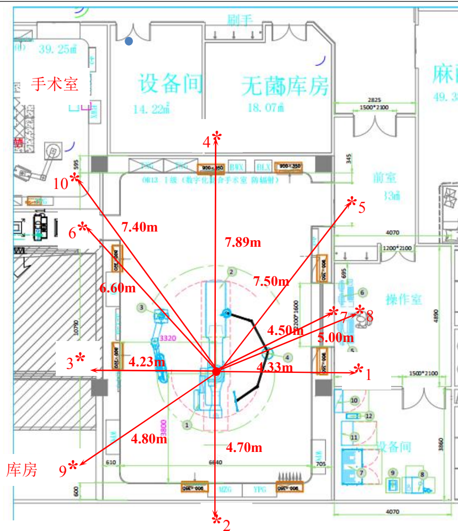
图 11-2 DSA机房所在楼层关注点位置
