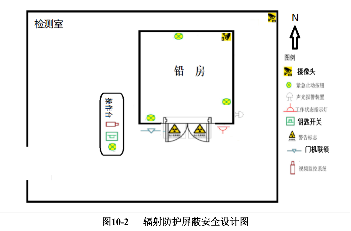
辐射防护屏蔽安全设计图 10-2。
