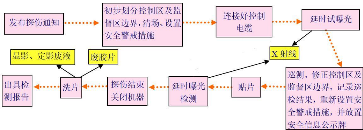
图 9-2 X 射线室外探伤工作流程及产污环节
