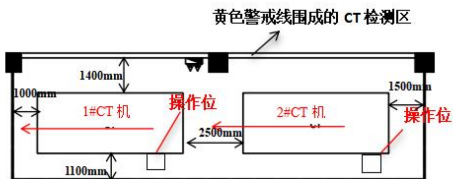
图 1.3-6.8 W22 厂房 2 层 1 号 CT 检测区平面布置图
