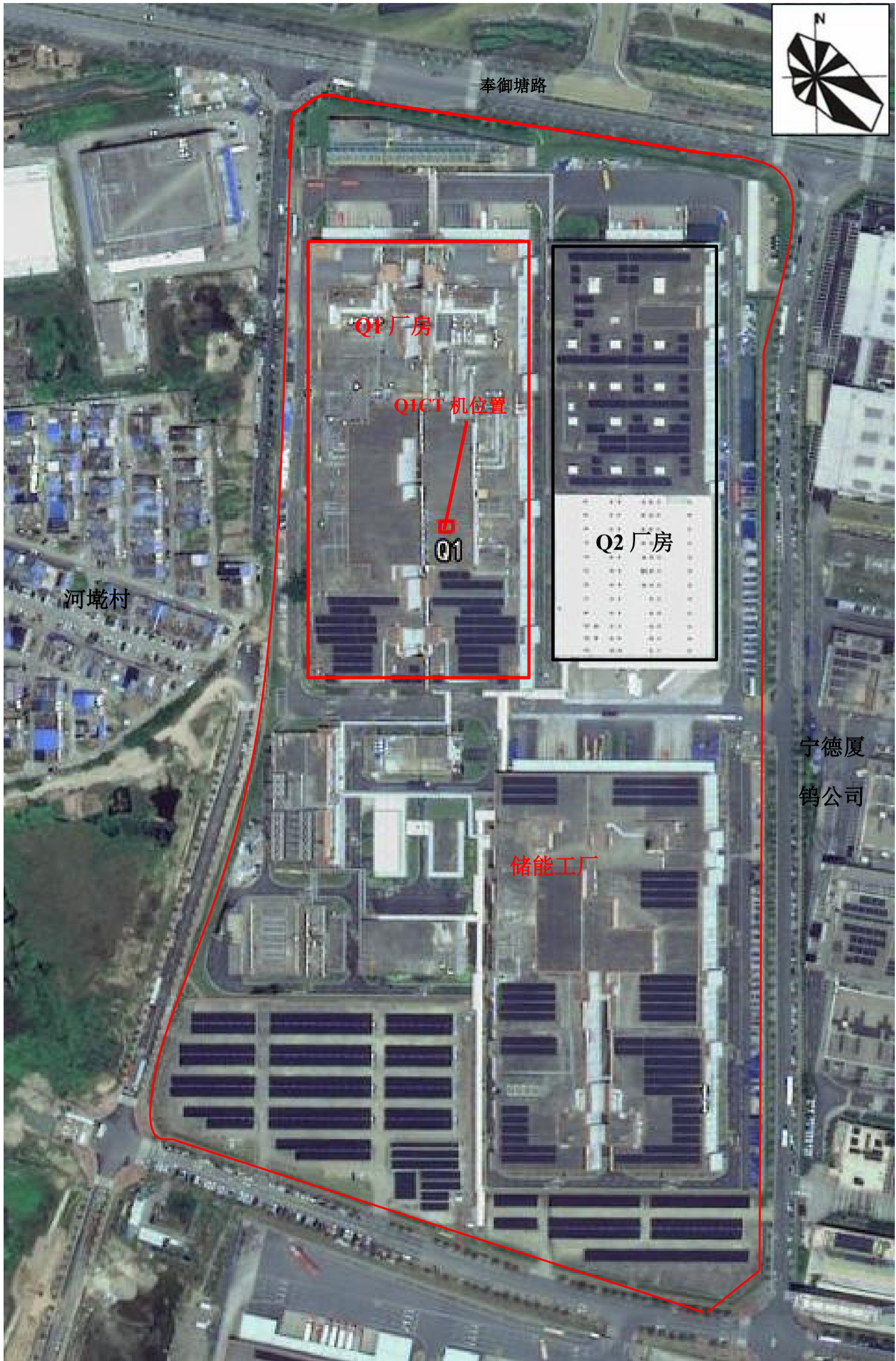
图 1-5.1 储能工厂平面布置图
