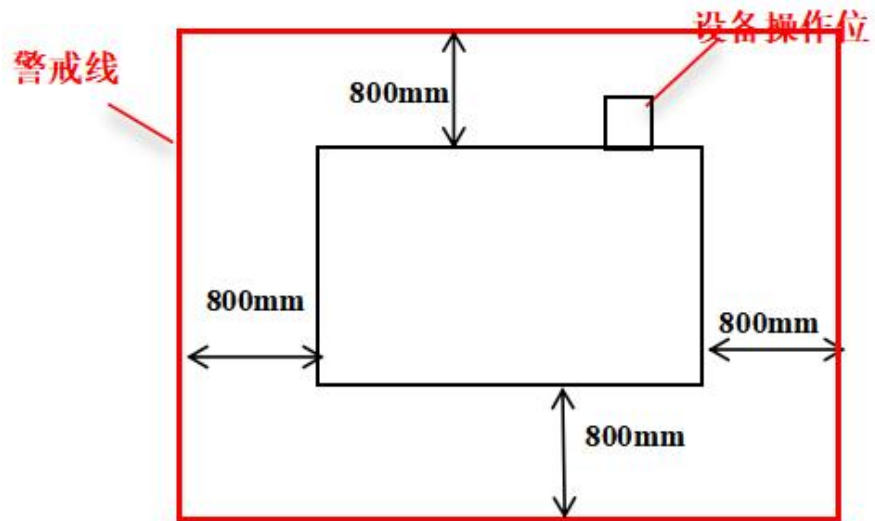
图 1-5.3 1 厂房 4 层 L81 拉线 CT 检测区平面布置图
