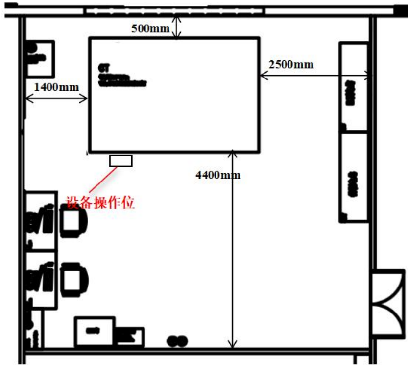
图 1-6.4 3号 CT 室平面布置图
