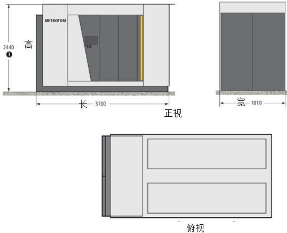
图 9-3 Z 基地 CT 机外部效果图
