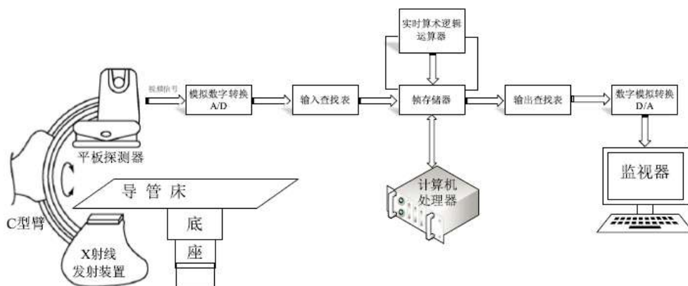
图 9-2 平板探测器型 DSA 机系统结构图
