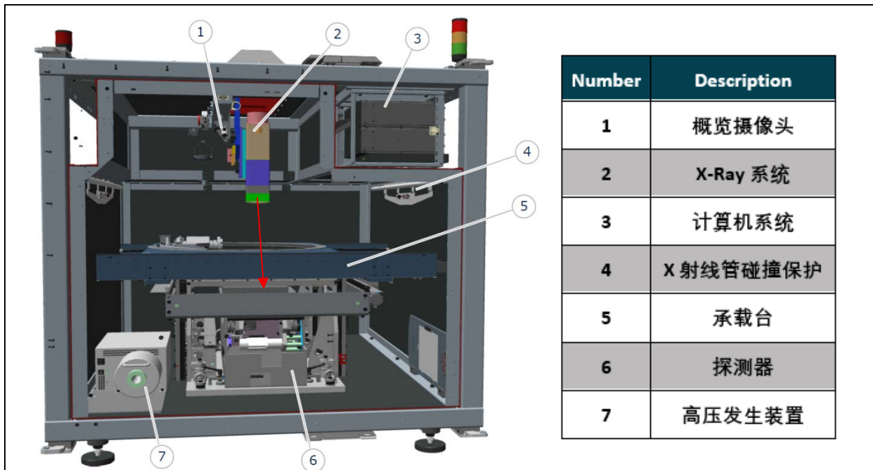
图 9.1 工业 CT 机设备结构示意图
