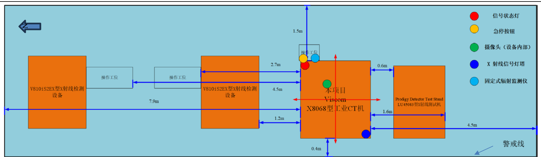
图 10.4 Viscom X8068 型防护装置示意图
