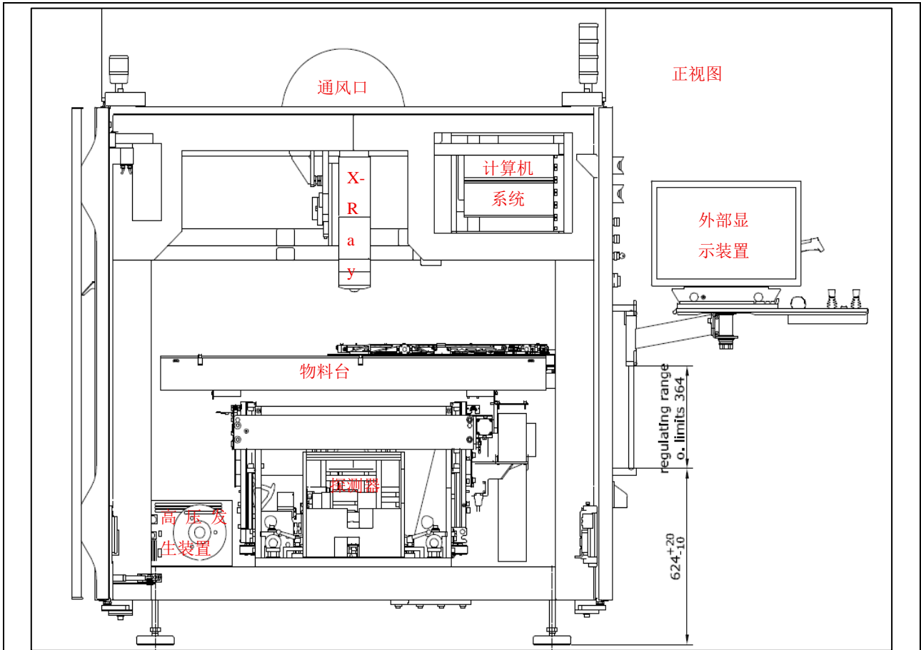
图 9.4 Viscom X8068 型工业 CT 机内部结构示意图
