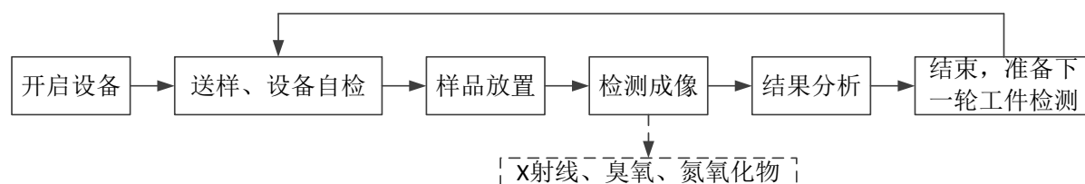
图 9.7 项目 X 射线数字成像系统工作流程及产污环节示意图
