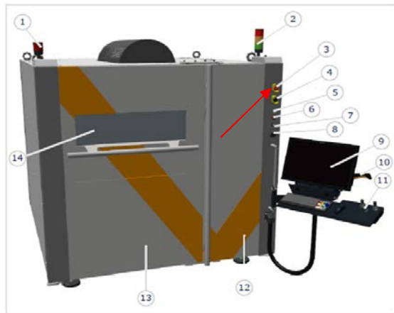
图 10.4 Viscom X8068 型防护装置示意图
