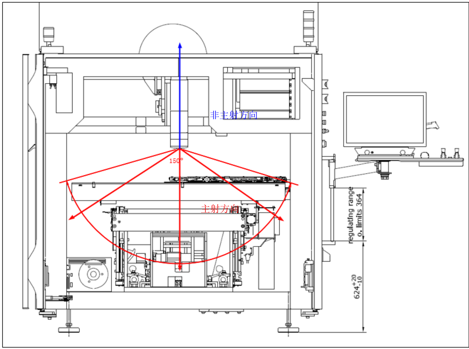
图 10.2 Viscom X8068 型工业 CT 机射线源方向示意（正向透视）
