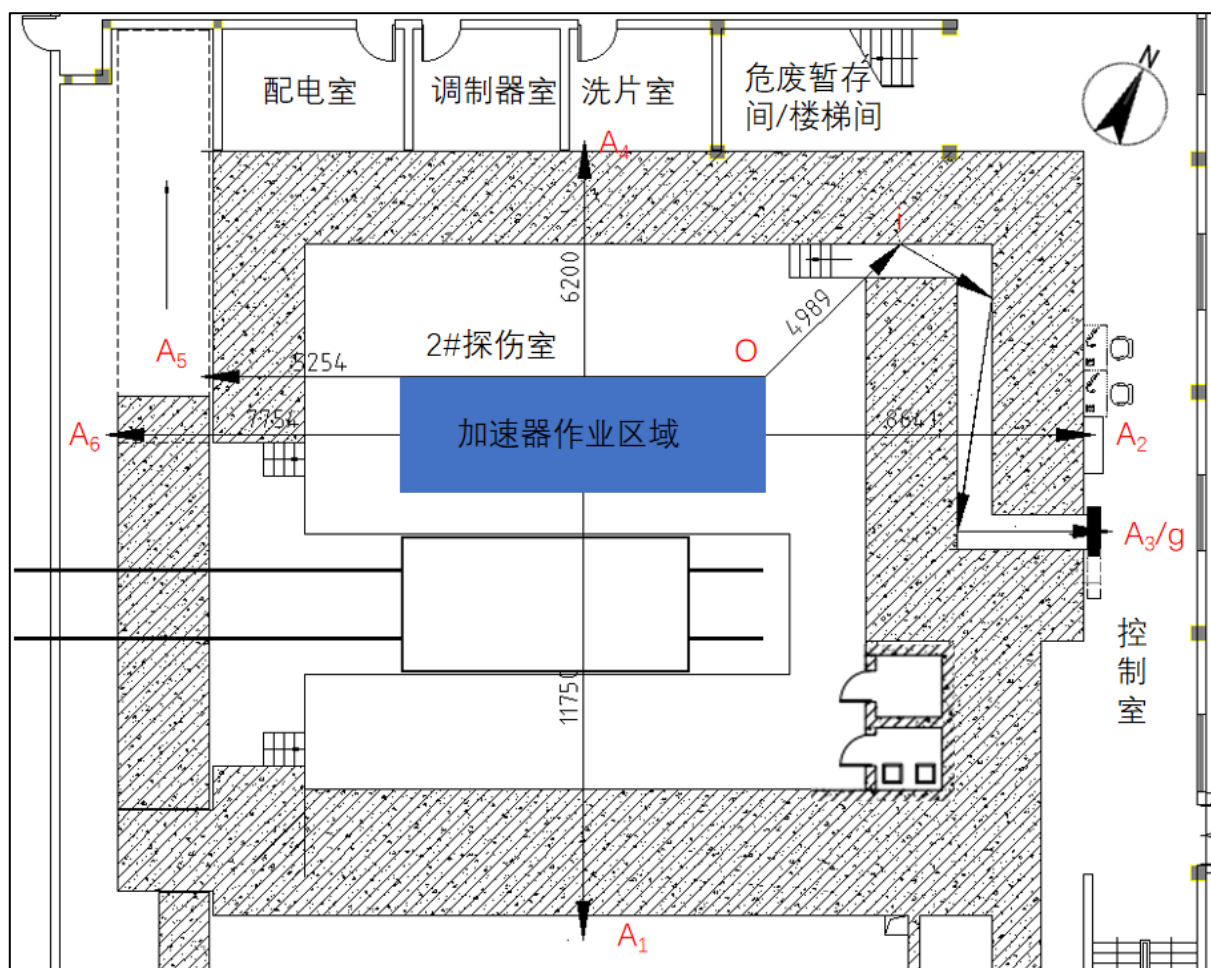
图 11-1 电子直线加速器预测点位平面示意图 (单位: mm)
