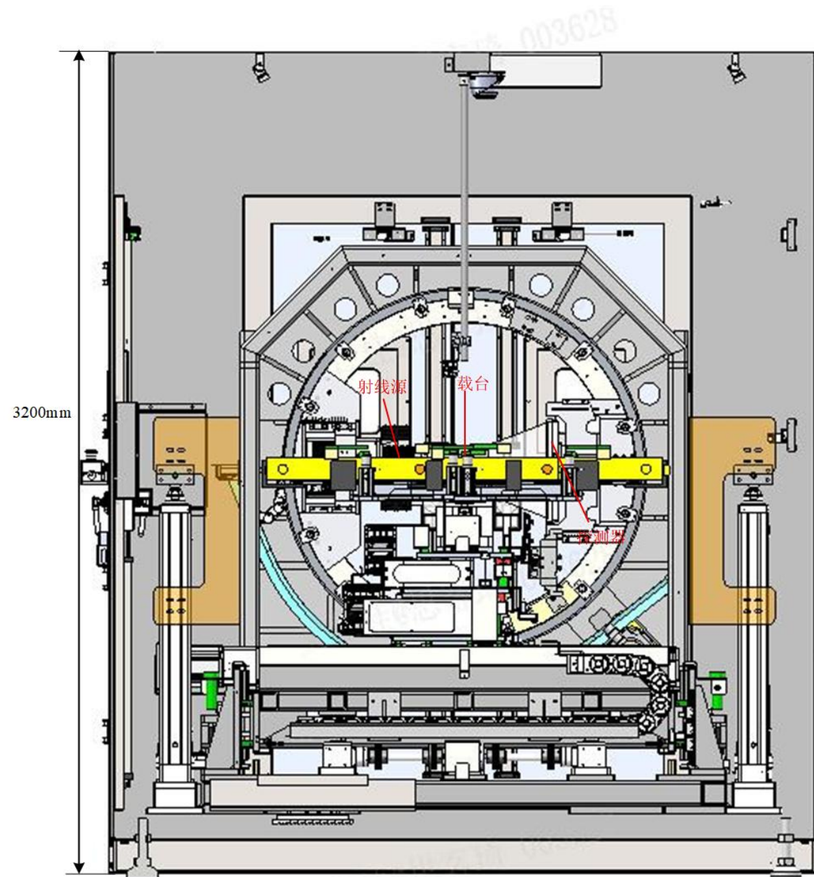
正视面
