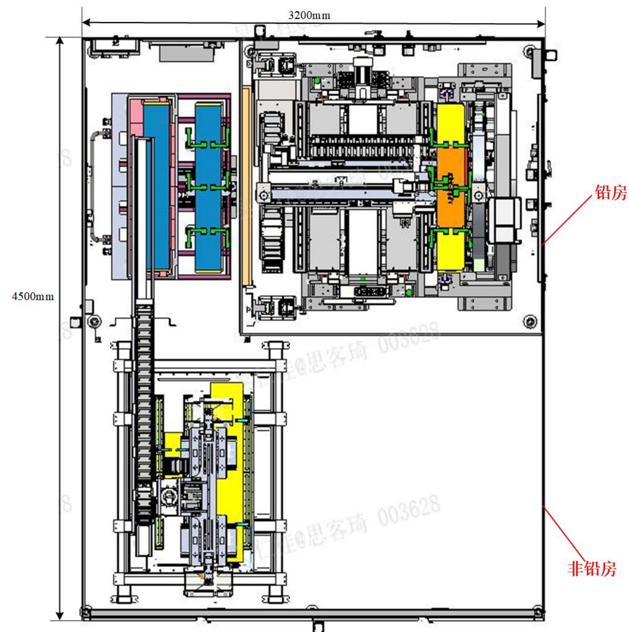
俯视面
