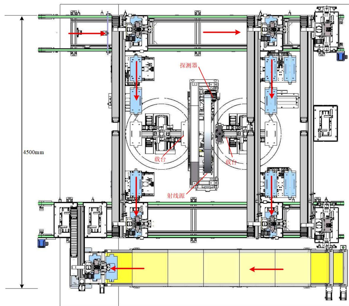
俯视面
