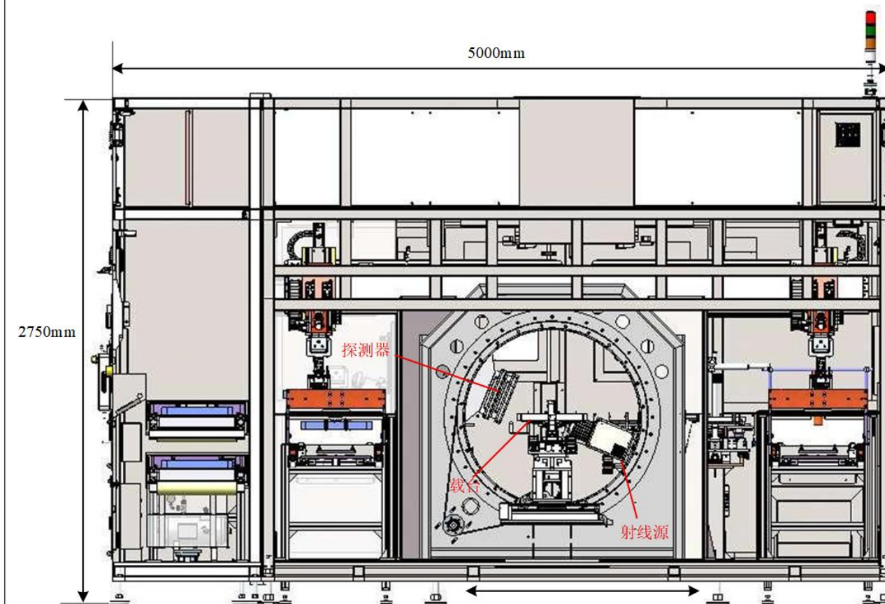
正视面
