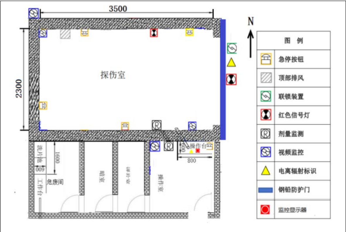
辐射防护屏蔽设计图 10-2。
