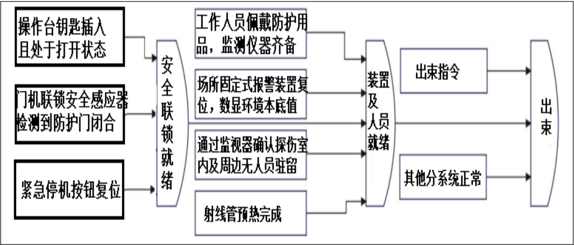
图10-4 辐射安全设施安全联锁逻辑图
