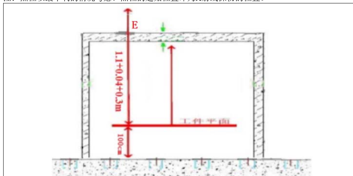
图11-2 剖面示意图（定向机）
