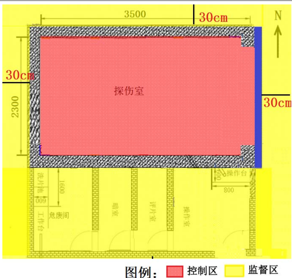
图10-1 本项目辐射工作场所分区示意图
