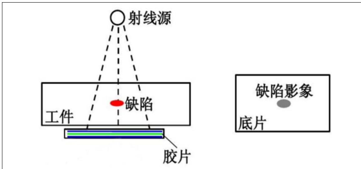
图9.1-3 X射线发生器工作原理示意图
