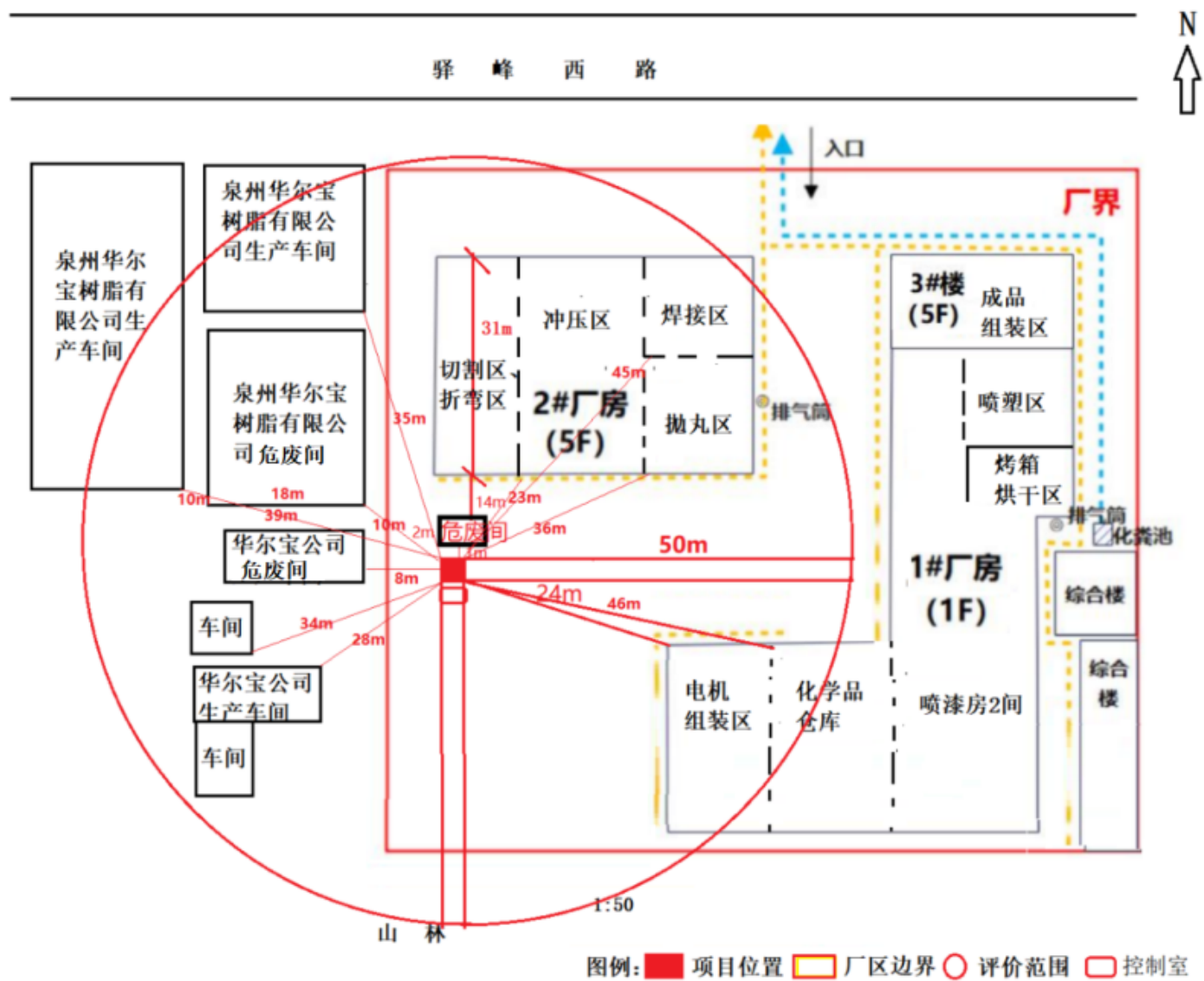
图 1.1-4 项目平面布置图
