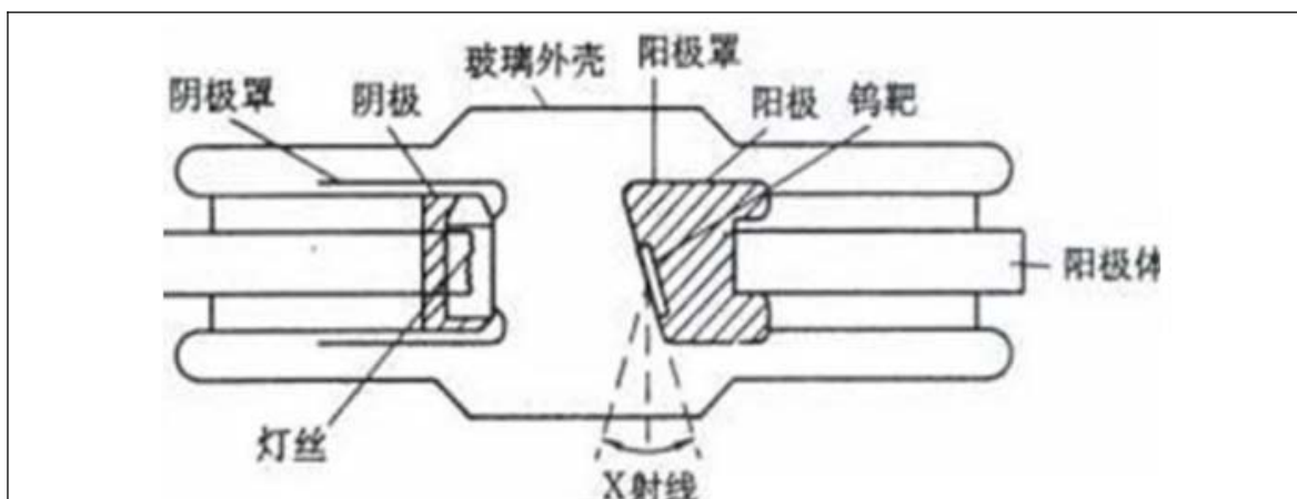
图9.1-2 X射线产生的示意图
