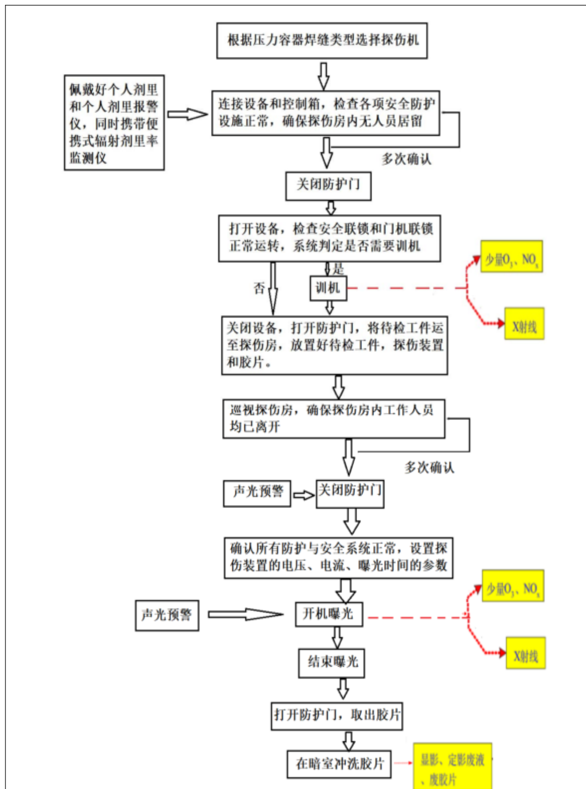
图 9.1-4 X 射线探伤机工艺流程图及产污环节示意图
